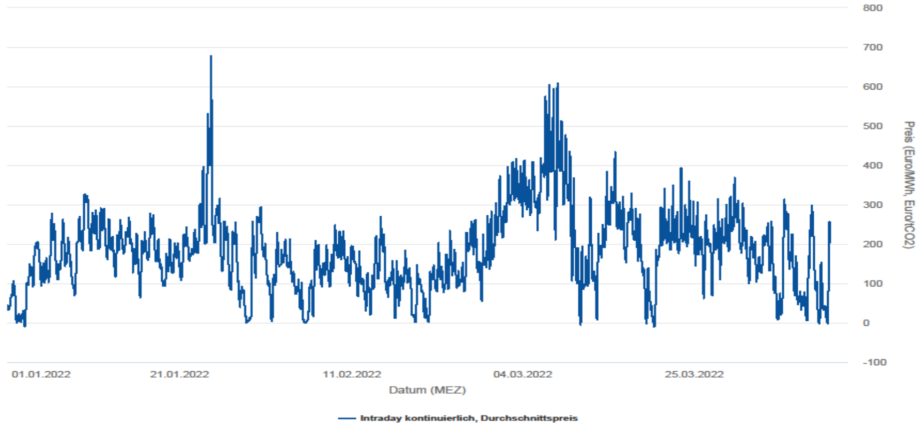
Stromproduktion und Börsenstrompreise in Deutschland 2022
